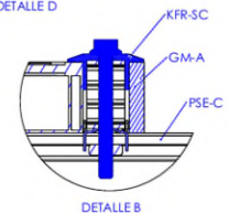
DETALLE B
