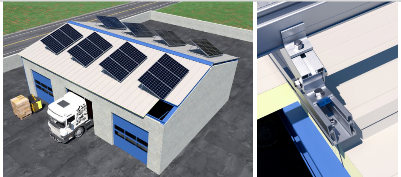
Beispiel 2: Dach mit gemischten Dachziegeln mit Sandwichpaneel / Befestigung mit Doppelgewindeschraube Metall KFS-AU
