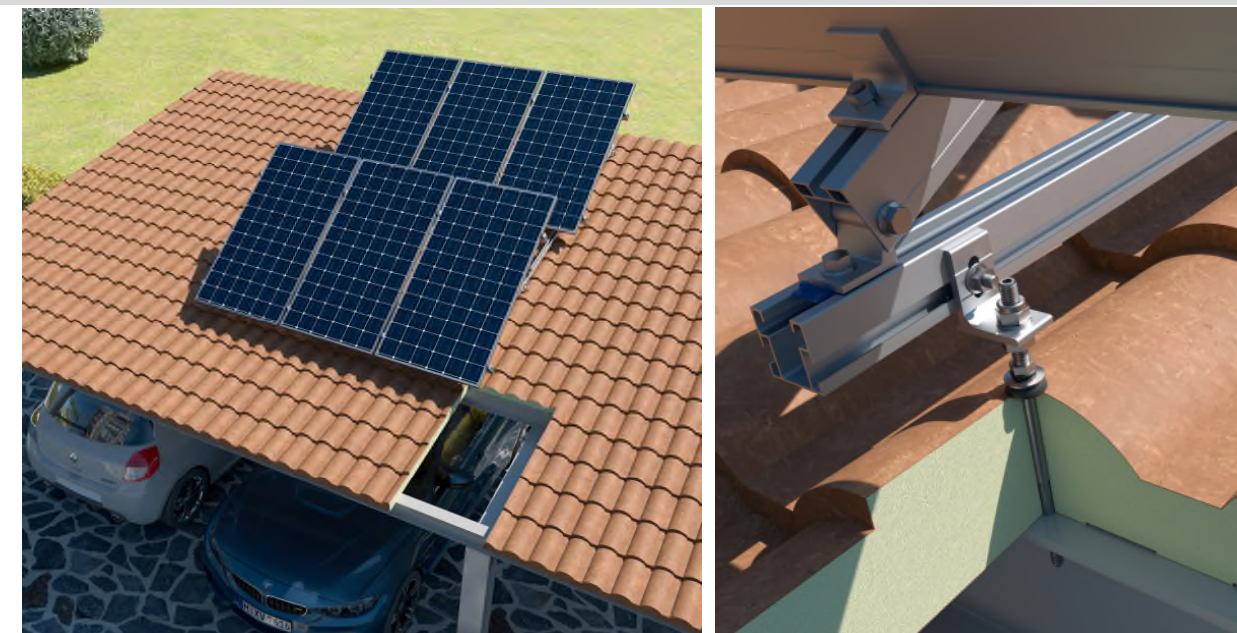
Beispiel 2: Dach mit gemischten Dachziegeln mit Sandwichpaneel / Befestigung mit Doppelgewindeschraube Metall KFS-AU
