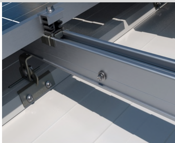
Ejemplo 2: Cubierta de panel sándwich 2 greclas con tapa juntas / fijación con soporte trapezoidal regulable STR
